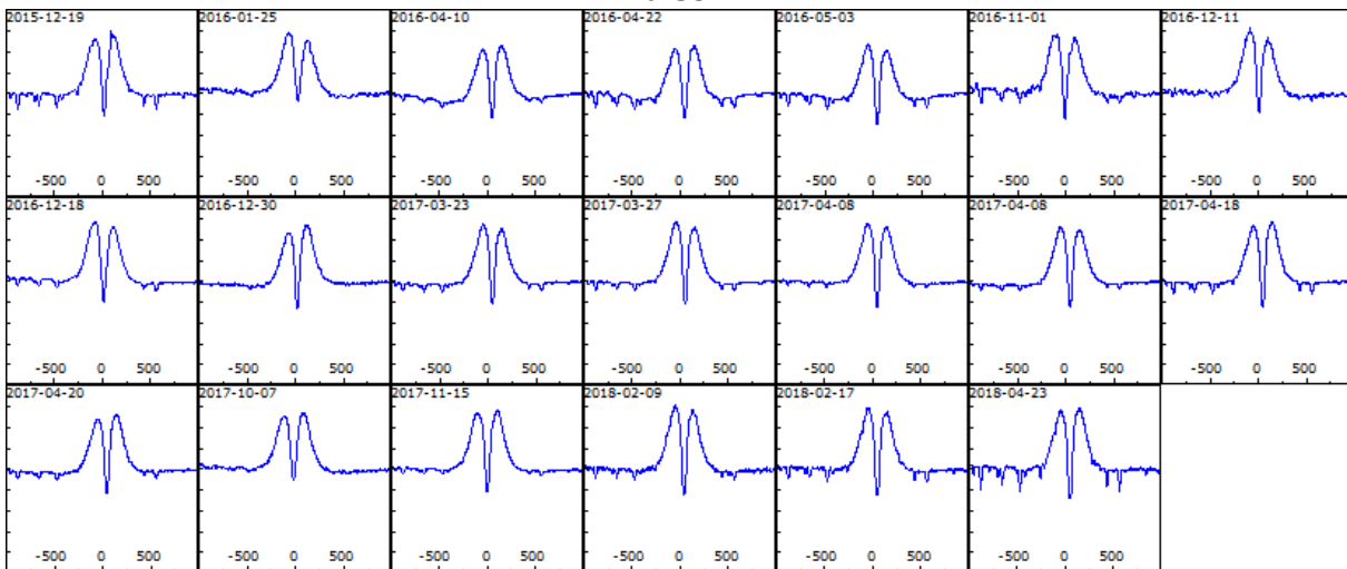
nu Gem
