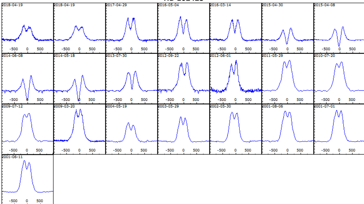
HD 162428
