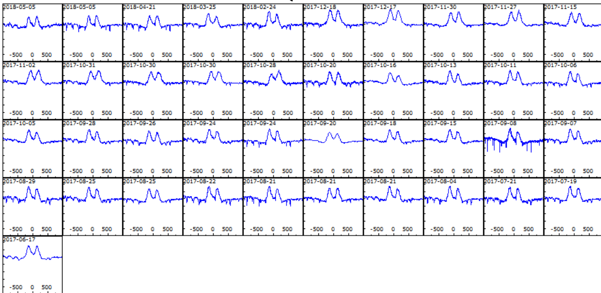
QR Vul
